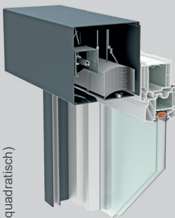
VORO PUTZ-90 (einputzbar)
