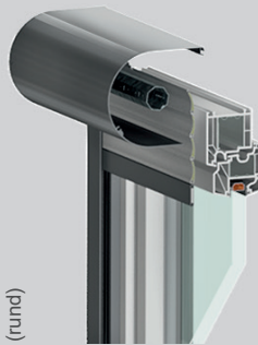
VORO SICHT-90 (quadratisch)
